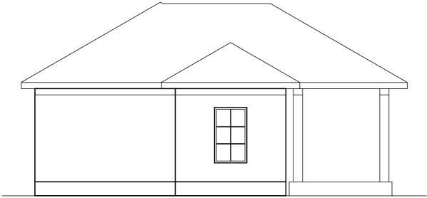
Elevación Lateral Derecha
