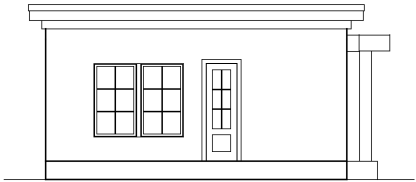
Elevación Lateral Izquierda
